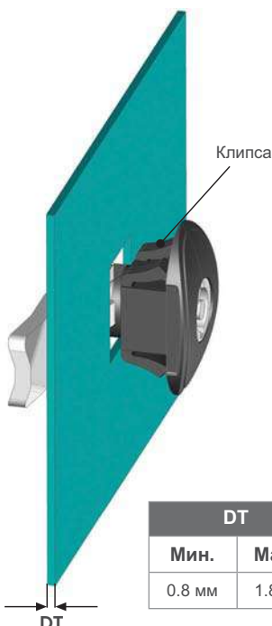
Толщина двери
