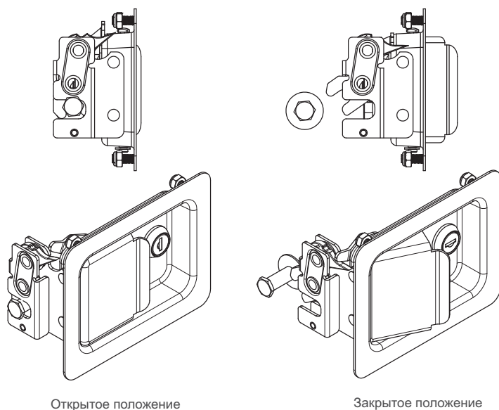
Открытое положение
