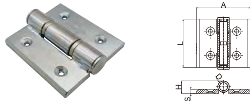
重型合页铰链 Folding Door Hinge
