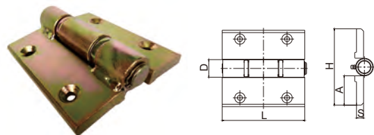
重型合页铰链 Folding Door Hinge
