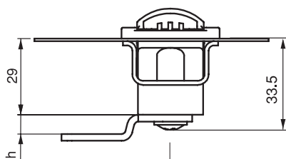
Стальной эксцентрик
