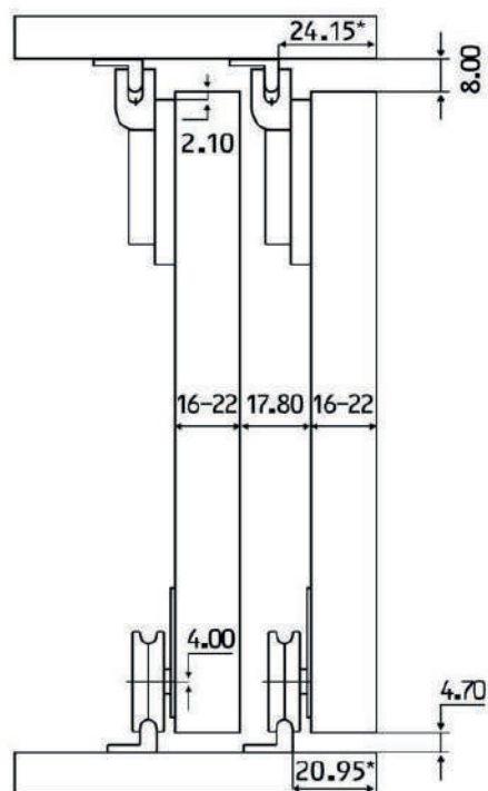
Мал. 2. Схема для розрахунків кріплення верхніх та нижніх профілів
