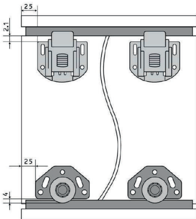
Мал. 1. Схема кріплення роликів
